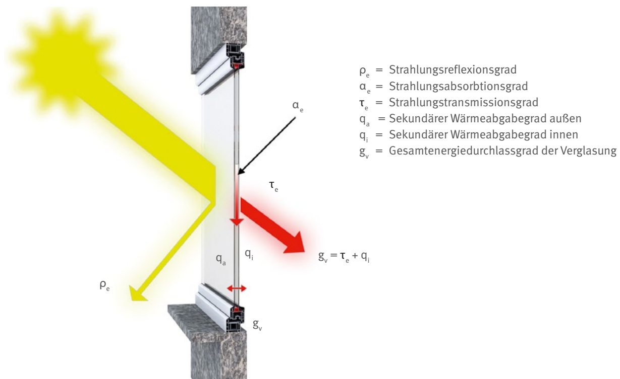
Abb. 3 Transmission, Reflexion, Absorption an einer Wärmeschutzverglasung
